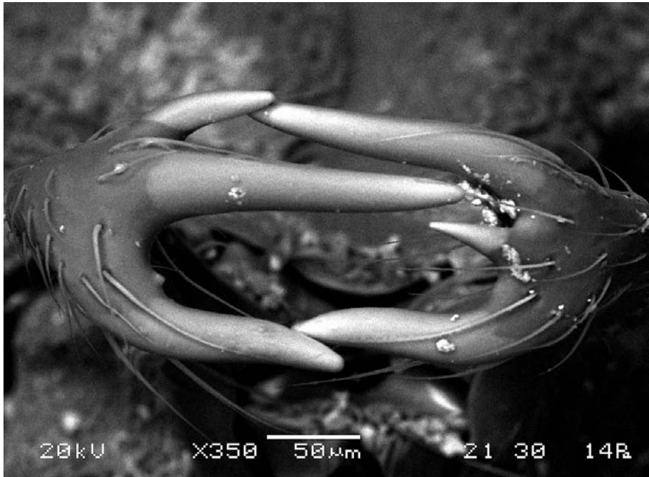
Fig. 3 - Strumigenys alessandrae n. sp., mandibular forks (apici delle mandibole).
