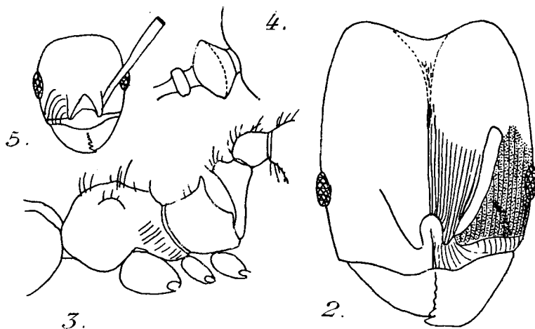
Fig. 2 à 5. — Pheidole hewitti , n. sp. Soldat : 2., tête; 3., thorax et pédoncule, de profil; 4., pédoncule vu de dessus. — Ouvrière : 5., tête.
