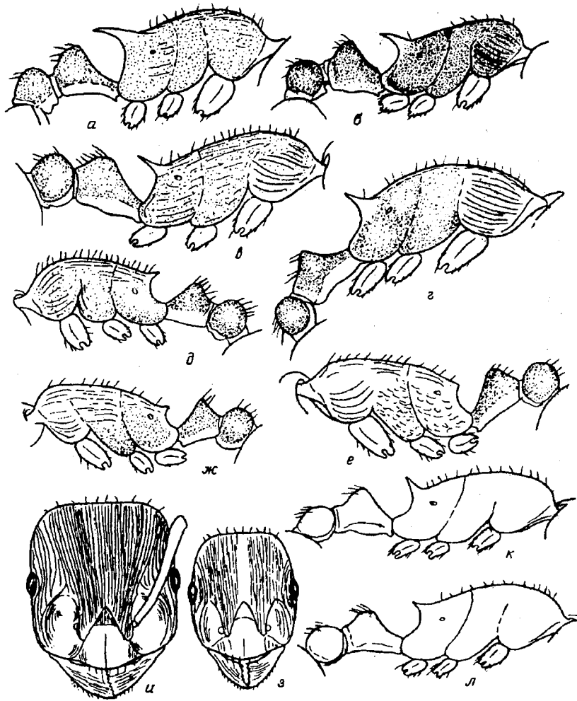
Рис. 7. Leptothorax nassonovi , неотип (а), L. knipovičschi , синтип (б), L. affinis (в), L. discoloratus , голотип (г), L. mongolicus , паратип (д), L. archangelskii , лектотип (е), L. tianshanicus , паратип (ж, з), L. corticalis (и), L. tauricus , неотип (к), L. unifasciatus (л): а — ж, к, л — грудь и стебелек в профиль; з, и — голова спереди (рабочие)
