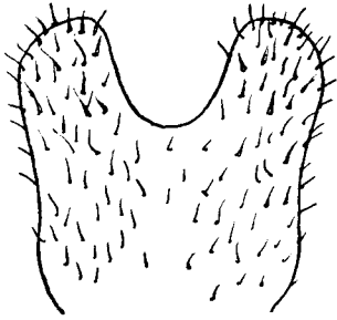
Abb. 7. Petiolus der Weibchen F. forsslundi Lohm. ssp. strawinski n. ssp.
