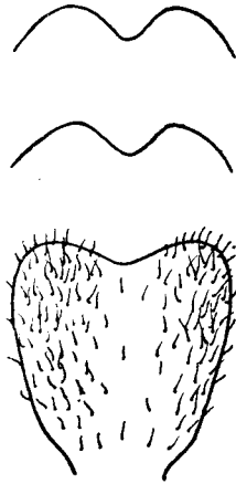
Abb. 11. Pet'olus der Arbeiterin F. forsslundi Lohm. ssp. strawinski n. ssp.
