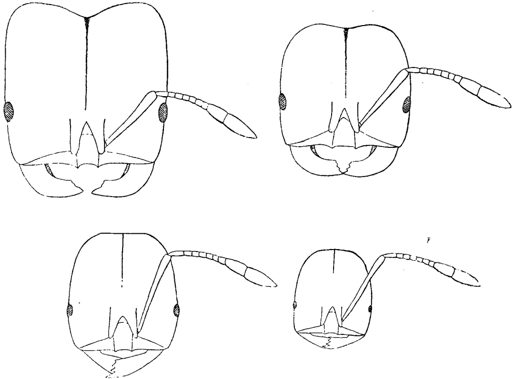
Fig. 4. — Solenopsis geminata F. — Capo delle diverse forme di operaie.
