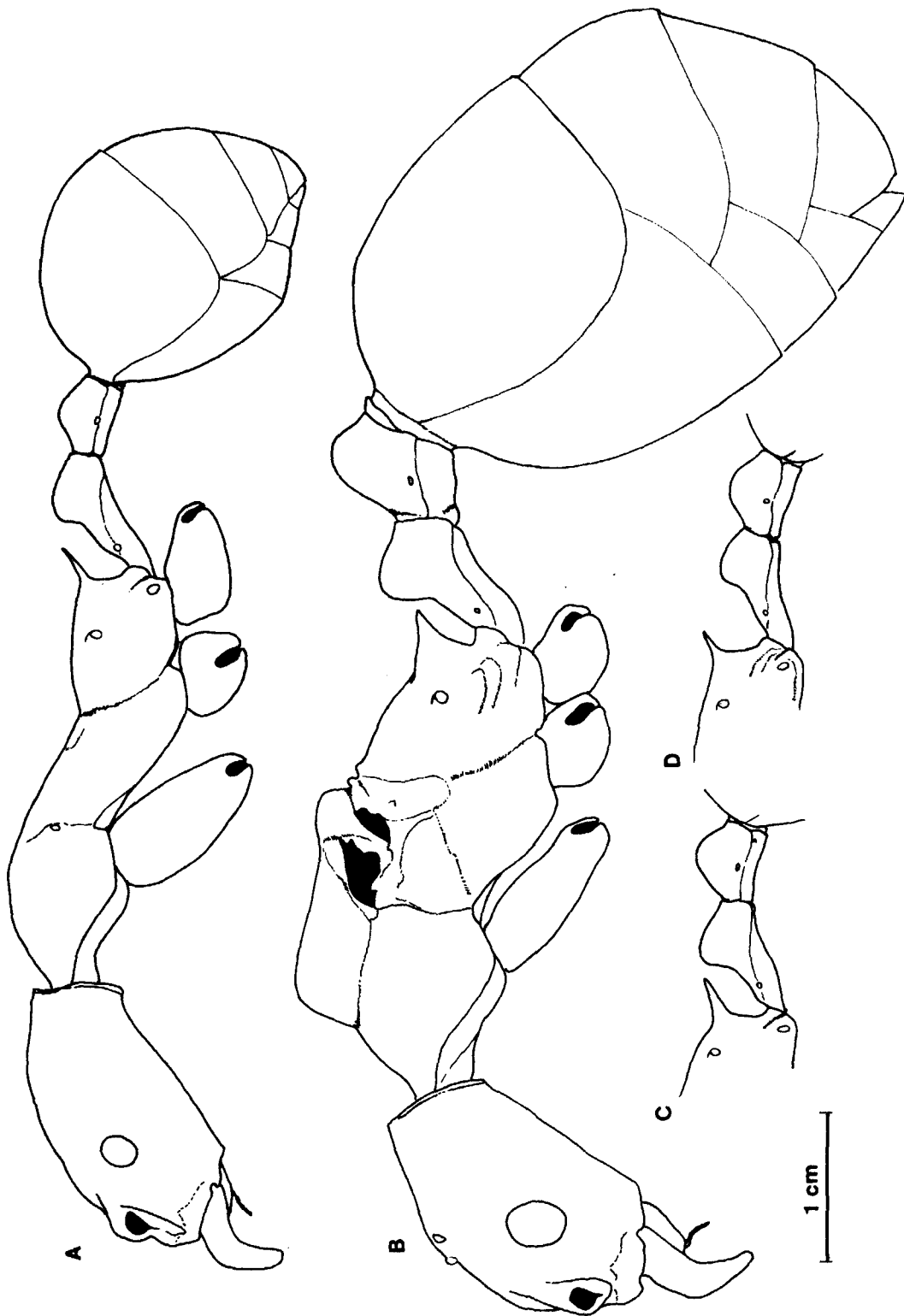
Fig. 2. — Aphaenogaster fallax sp. n. Profil d'une ouvrière du Todra, Maroc (A). profil d'une reine, même provenance (B). Profil du propodéum et des pétioles d'une ouvrière de Tammarakech, gorges du Ziz, Maroc (C). Idem d'une ouvrière du Djebel Mzi, Algérie (D).
